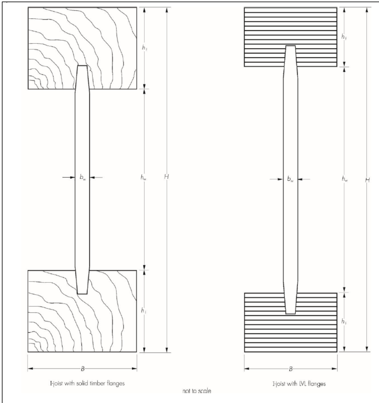
Abbildung A1 Querschnitte (Abmessungen in mm)
