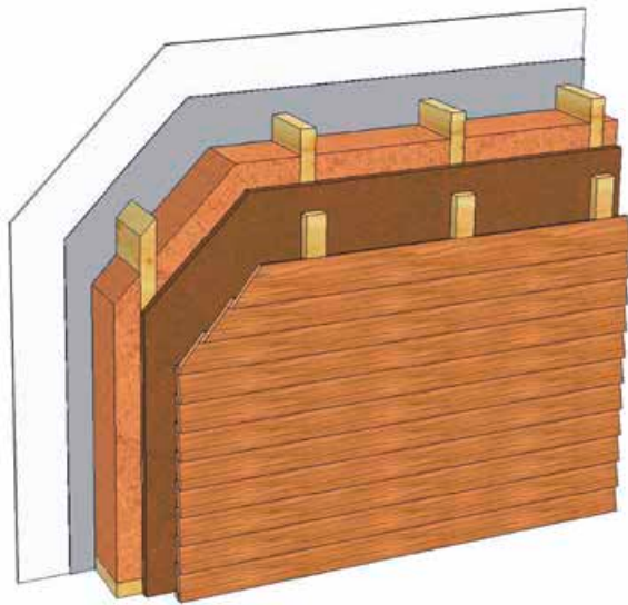
Produktblatt STEICO duo dry
