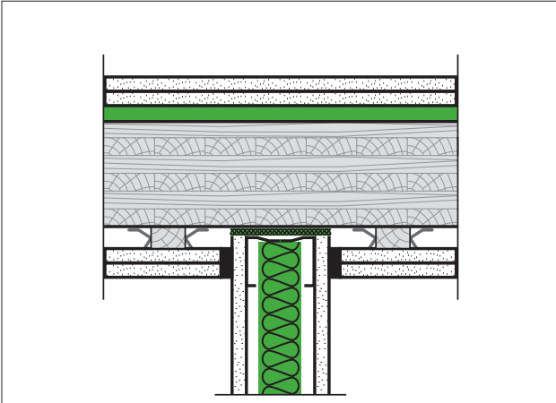
| ANSCHLUSS AN MASSIVHOLZDECKE
