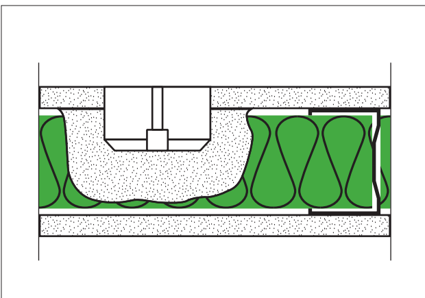
| BRANDSCHUTZTECHNISCHER EINBAU STECKDOSE MIT GIPSMÖRTEL
